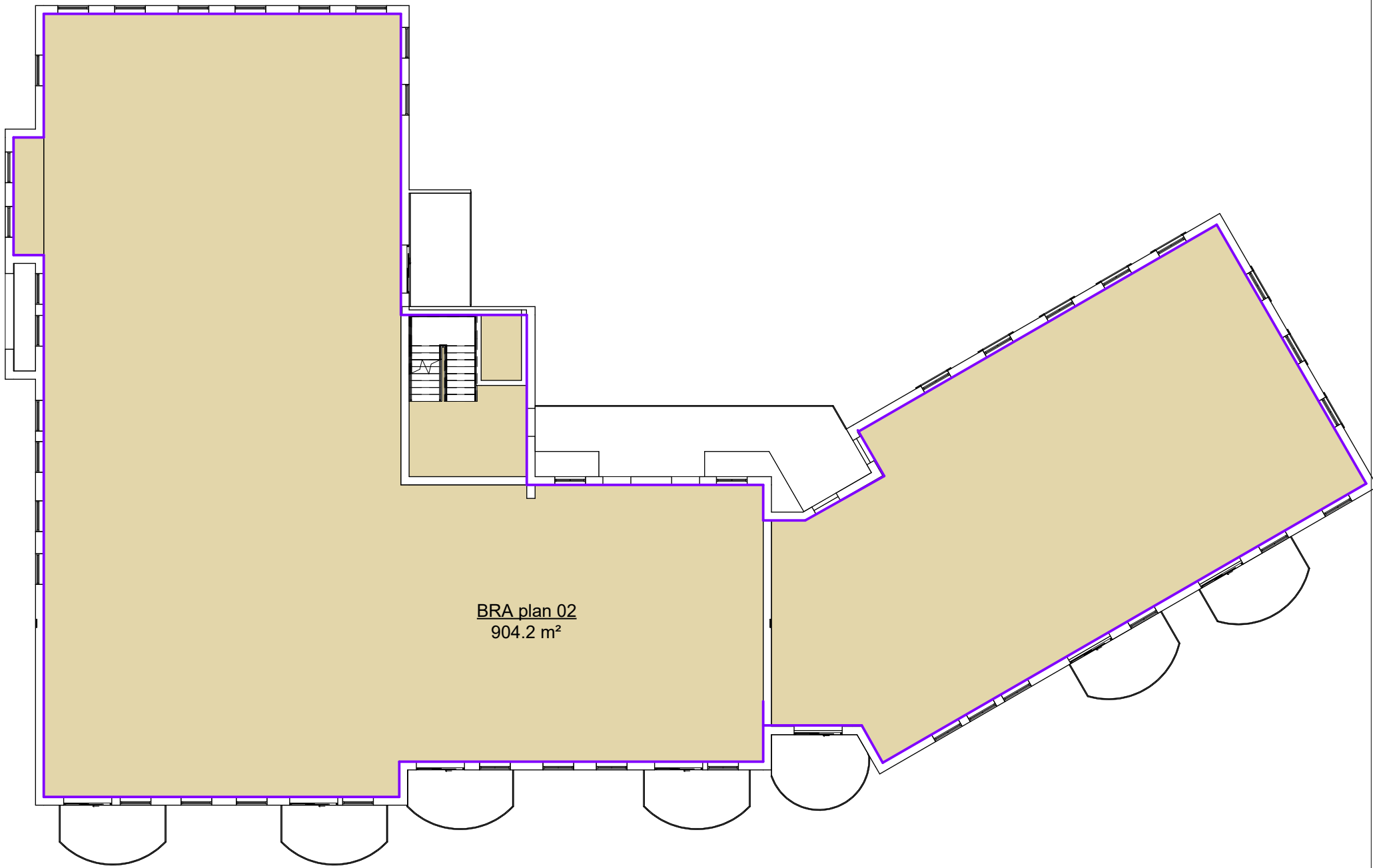
2 Plan 02 1 : 200
