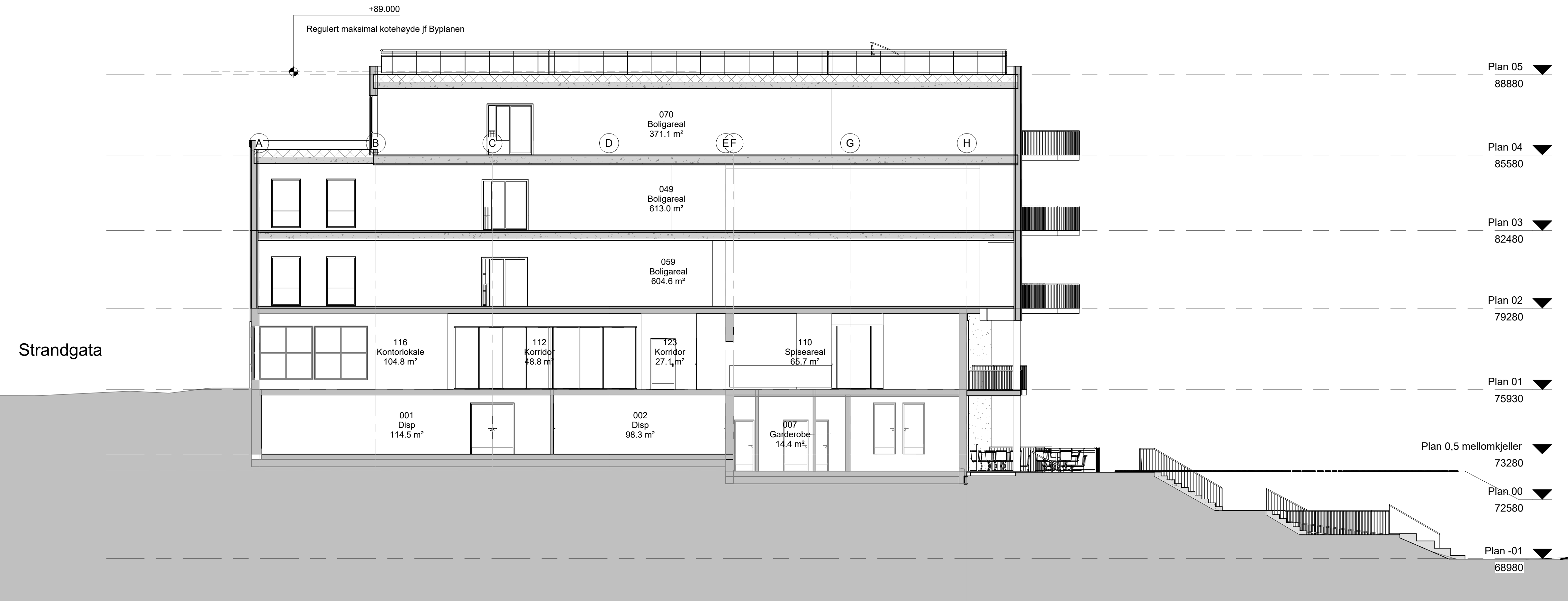
2 Snitt B 1 : 100
