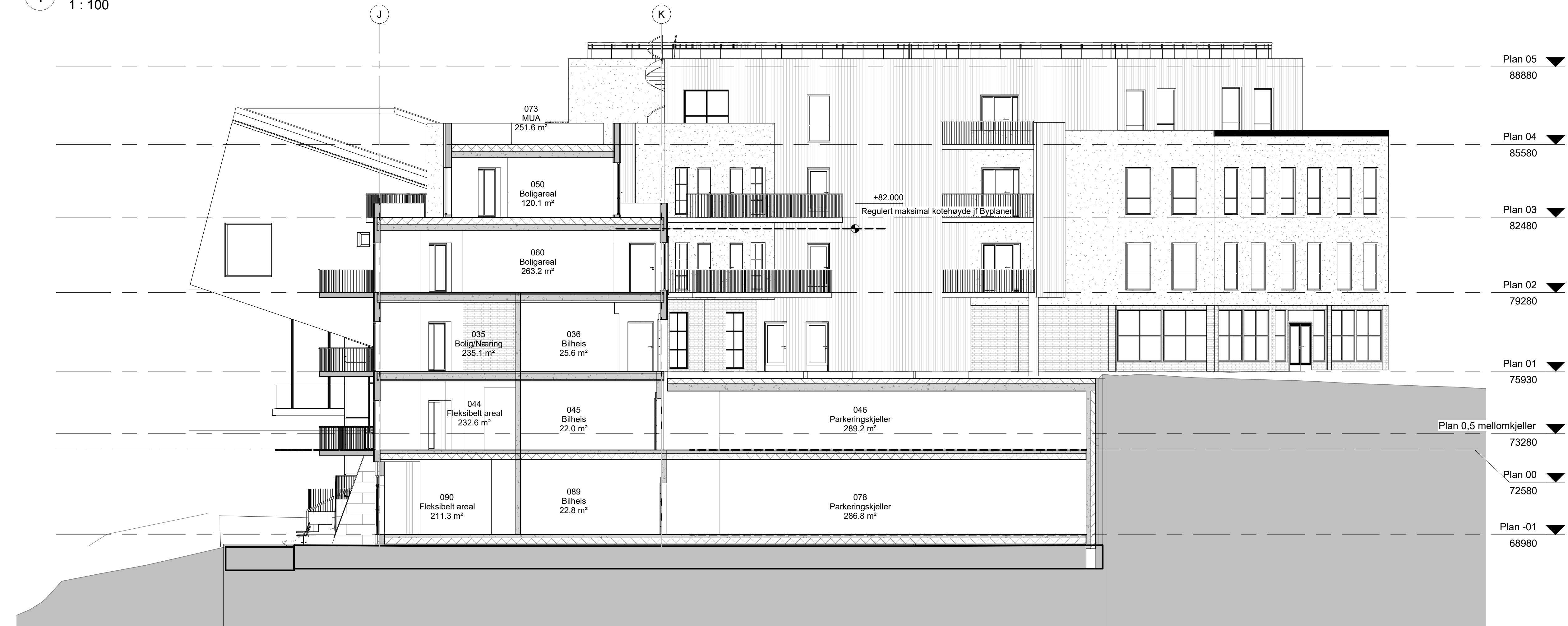
2 Snitt D 1 : 100
